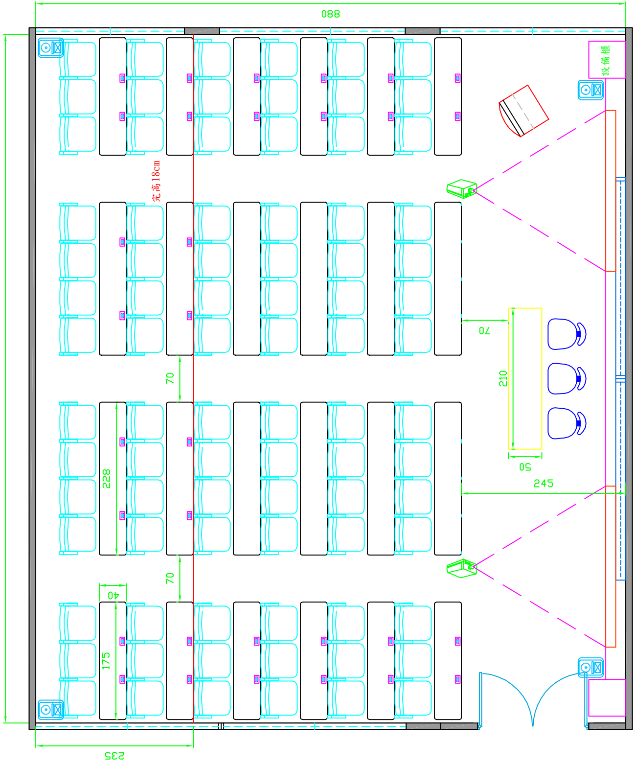
管3015教室規畫平面圖(84人座)
